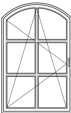
Okno se segmentovým obloukem OS s příčlemi v křídle
