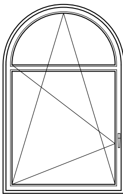
Okno s půlkruhovým obloukem OS s příčlím v křídle
