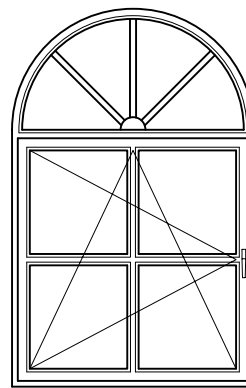
Okno s půlkruhovým obloukem OS s příčlemi v křídle a pevným nadsvětlíkem
